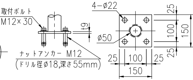
ベースプレート詳細図 (1/10)
