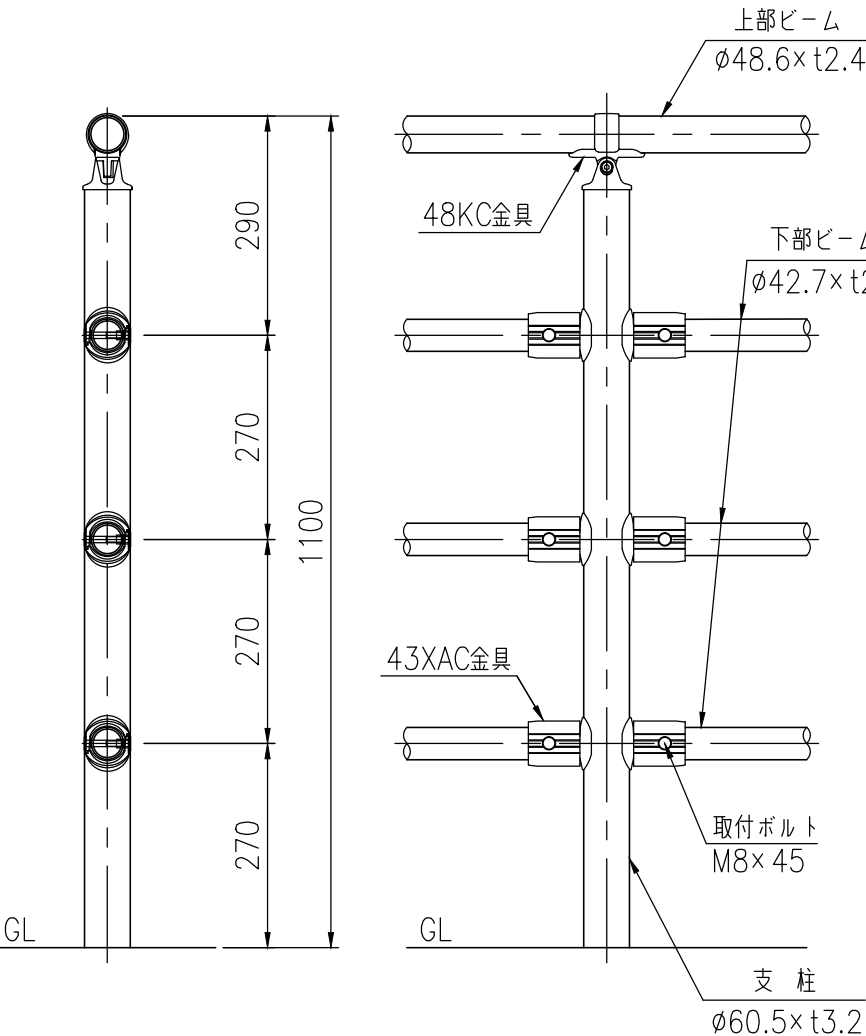
支柱図 (1/10)
