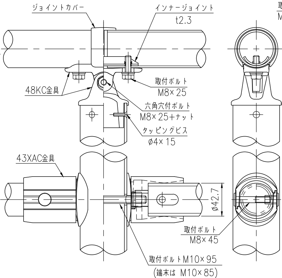
取付部詳細図 (1/3)
