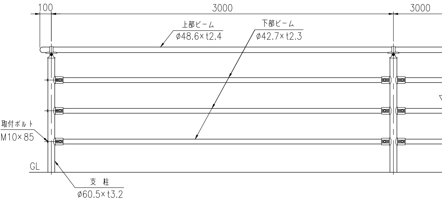
設置図 (1/20)
