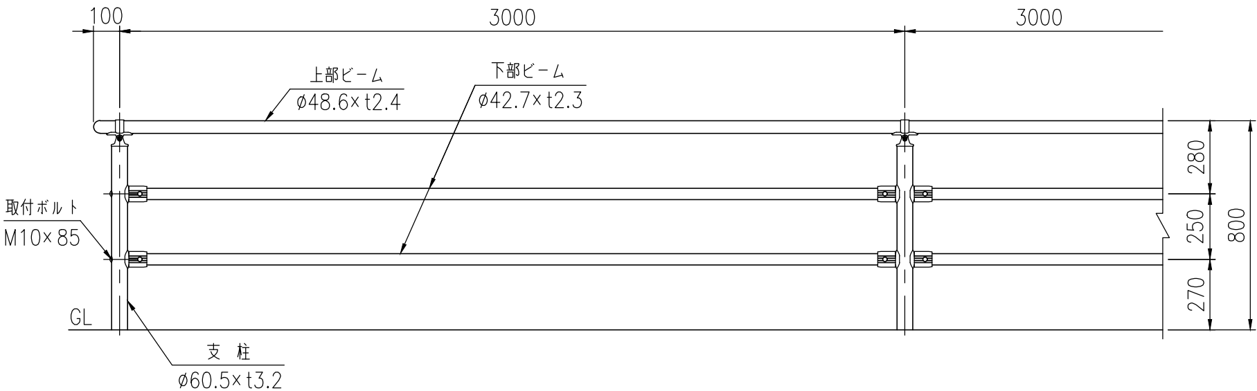
設置図 (1/20)
