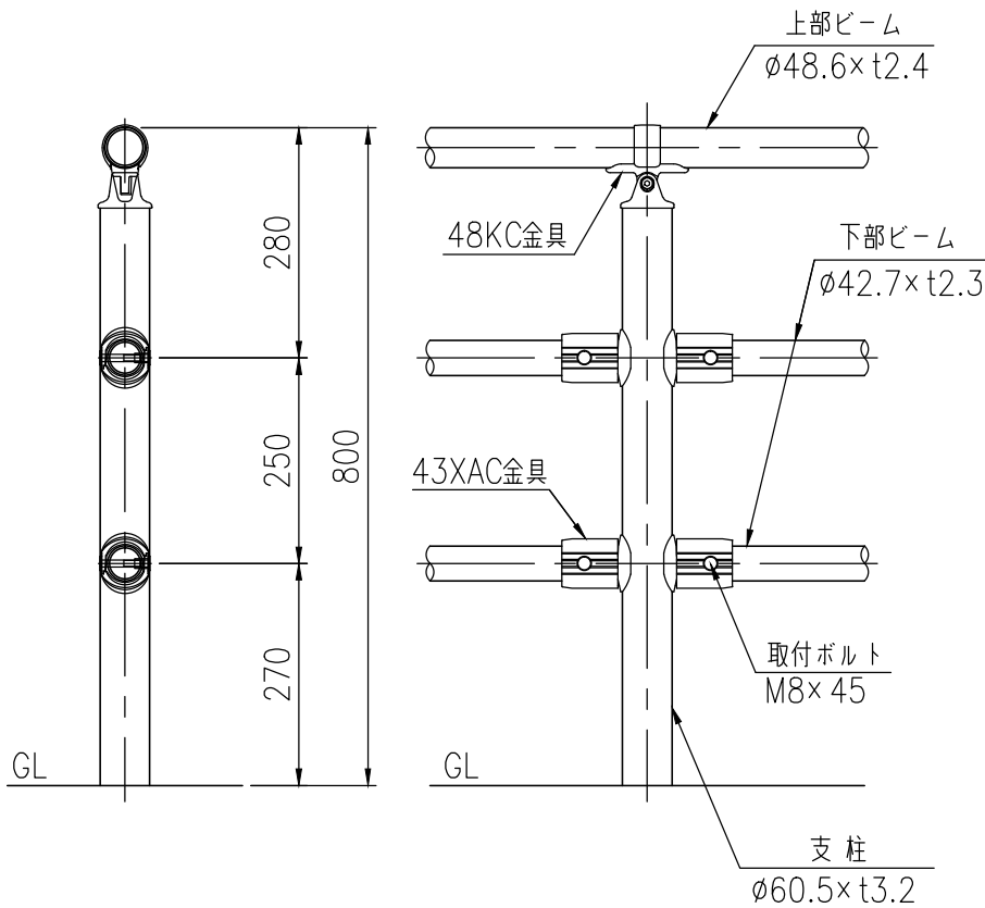
支柱図 (1/10)
