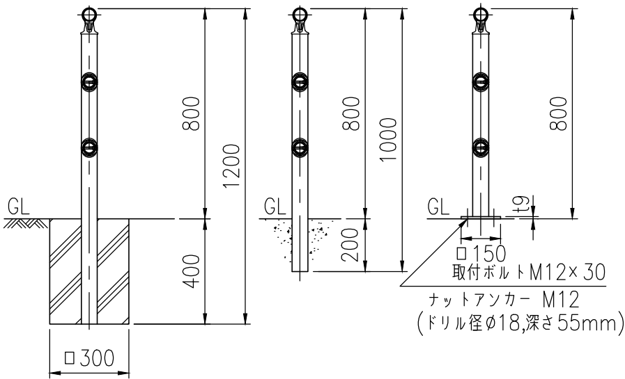
ベースプレート詳細図 (1/10)
