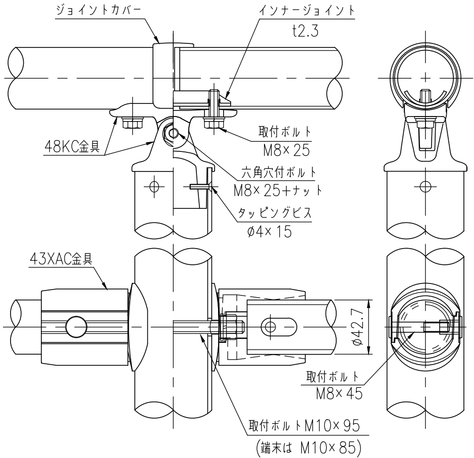
取付部詳細図 (1/3)
