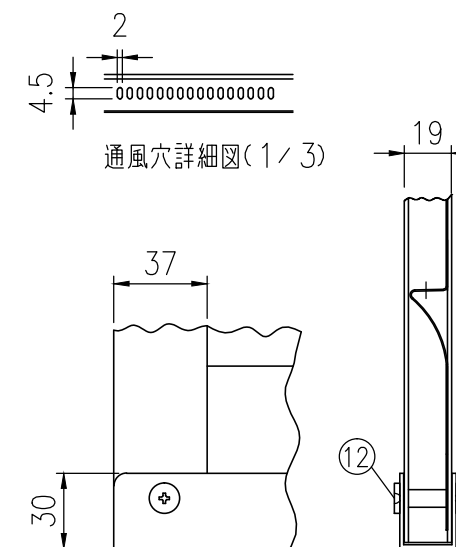
C部詳細図 (1/3)
