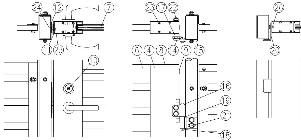
イ部詳細図 (1/8)
