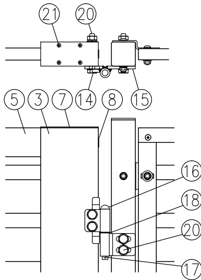
ロ部詳細図 (1/8)
