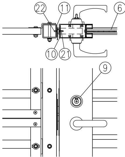
イ部詳細図 (1/8)
