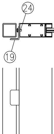
ハ部詳細図 (1/8)
