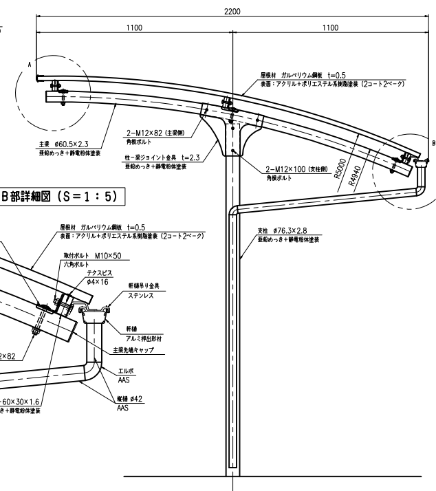
断面図 (S = 1 : 10)
