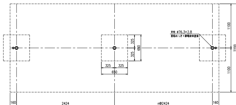
割付図 (S=1:20)
