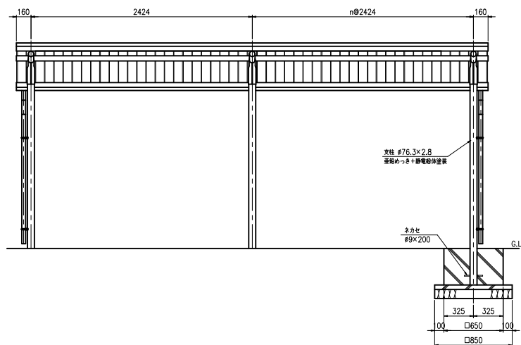
正面图 (S=1:20)
