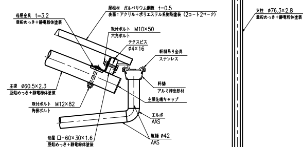
B部詳細図 (S = 1 : 5)
