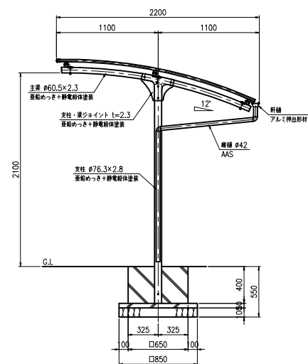
側面図 (S=1:20)
