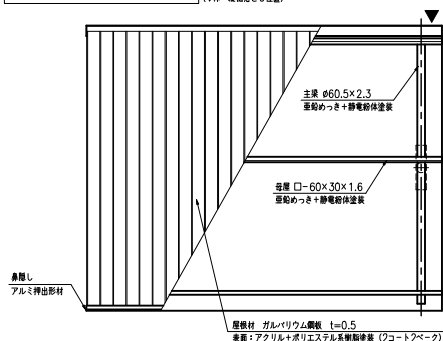
正面図 (S=1:20)
