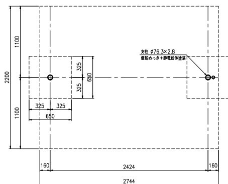
平面図 (S=1:20)
