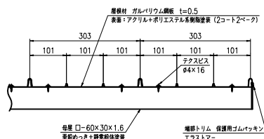
屋根材取付詳細図 (S=1:5)
