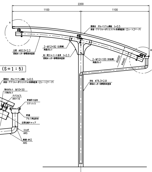
断面図 (S=1:10)
