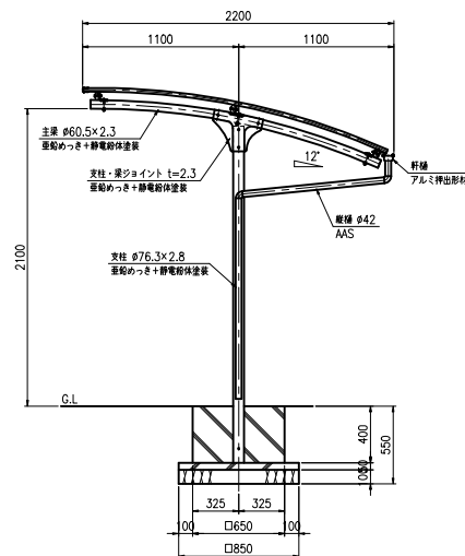
側面図 (S=1:20)
