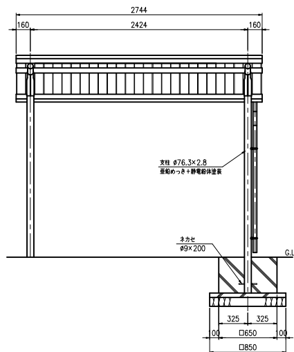
正面図 (S=1:20)
