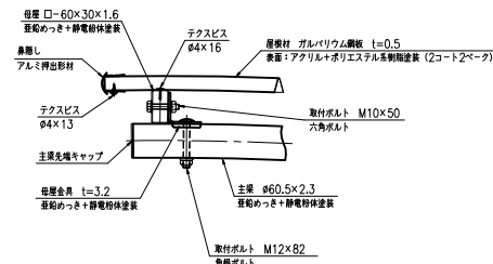
A部詳細図 (S=1:5)
