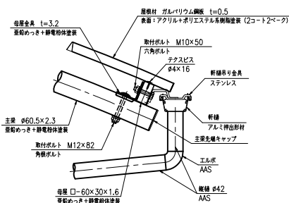
B部詳細図 (S=1:5)
