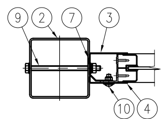
C-C 断面図 (1/8)
