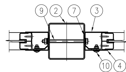
D-D 断面図 (1/8)
