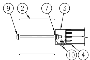
C-C 断面図 (1/8)
