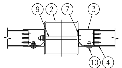
D-D 断面図 (1/8)
