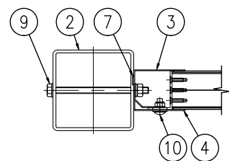
C-C 断面図 (1/8)
