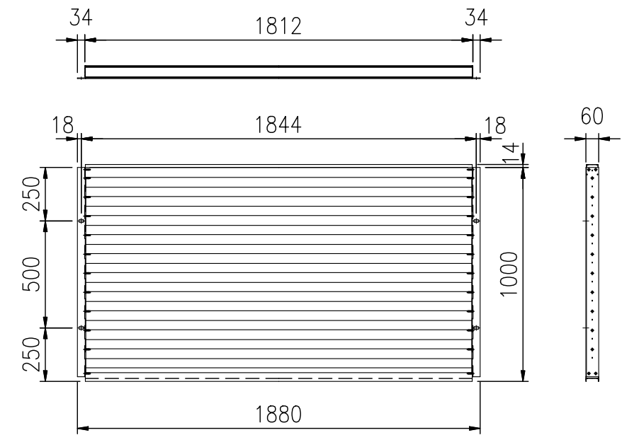
パネル H1m 詳細図 (1/25)
