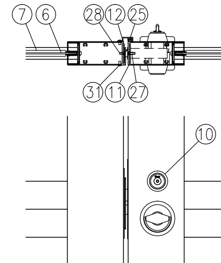
イ部詳細図 (1/8)
