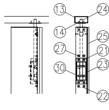
二部詳細図 (1/10)
