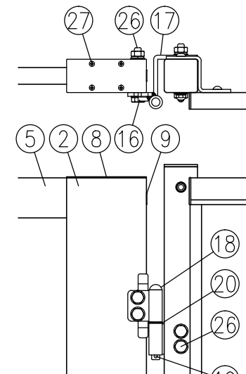
ロ部詳細図 (1/8)
