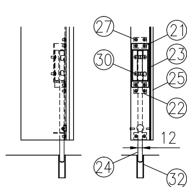
ハ部詳細図 (1/10)
