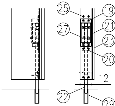
ハ部詳細図 (1/10)
