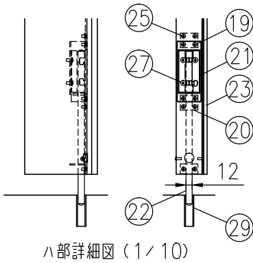
ハ部詳細図 (1/10)
