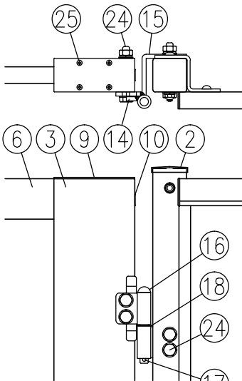
□部詳細図 (1/8)
