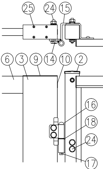
□部詳細図 (1/8)
