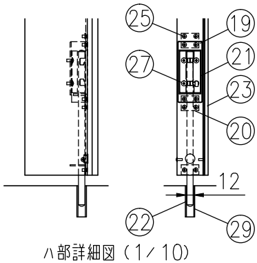
ハ部詳細図 (1/10)
