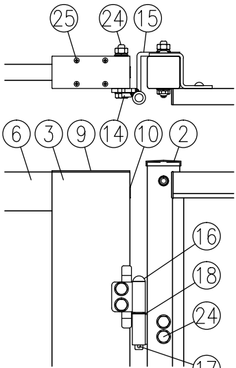
ロ部詳細図 (1/8)
