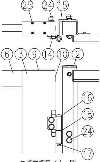
□部詳細図 (1/8)
