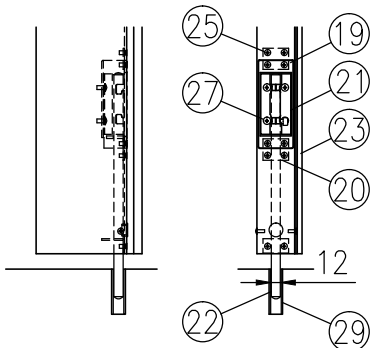
ハ部詳細図 (1/10)
