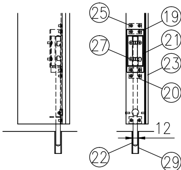
H部詳細図 (1/10)
