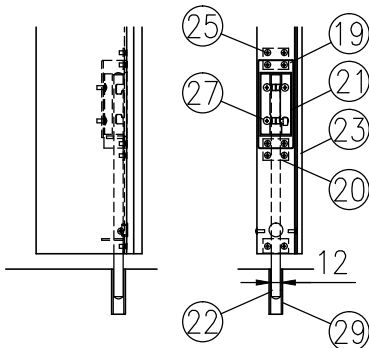
ハ部詳細図 (1/10)
