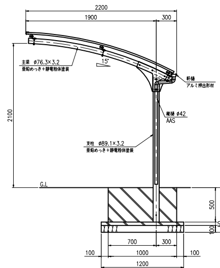
側面図 (S=1:20)
