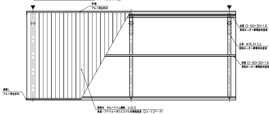
正面図 (S=1:20)
