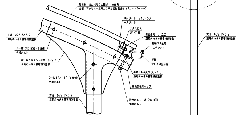
B部詳細図 (S=1:5)
