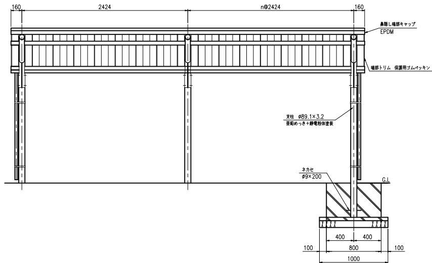
正面図 (S=1:20)
