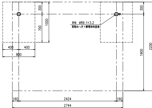
基礎伏図 (S=1:20)
