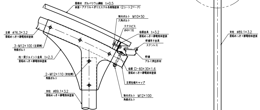
B部詳細図 (S=1:5)
