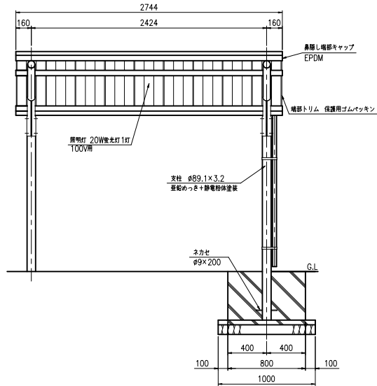
正面図 (S=1:20)
