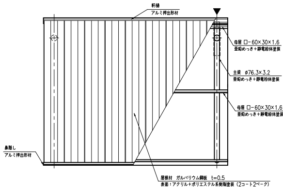
正面図 (S=1:20)
