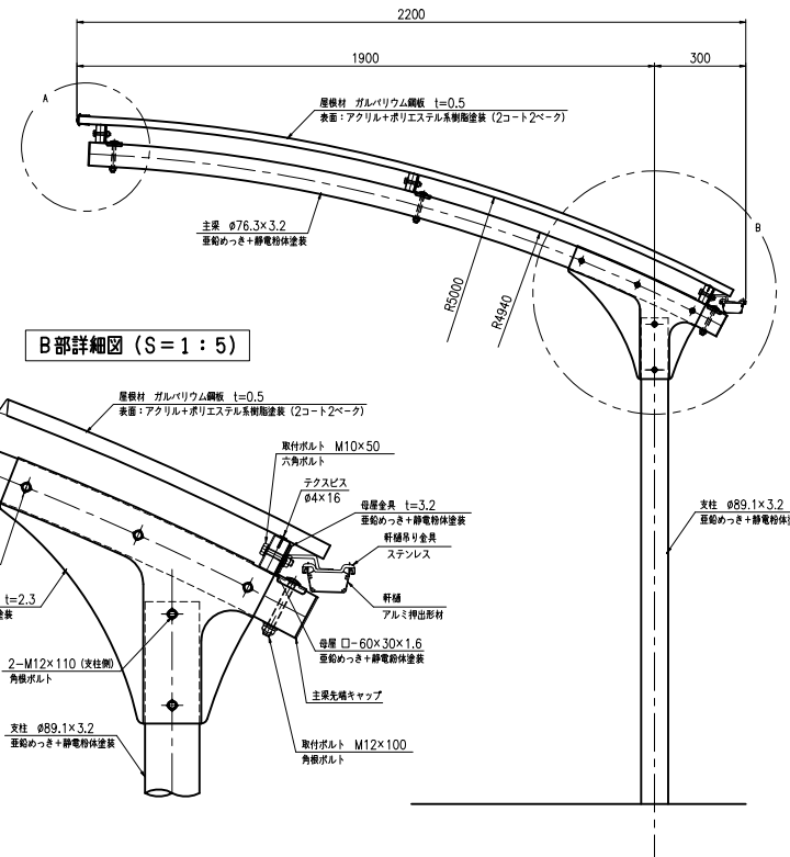
断面図 (S=1:10)
