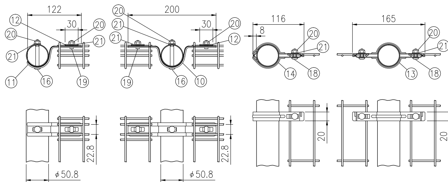
C部詳細図 (1/5)
