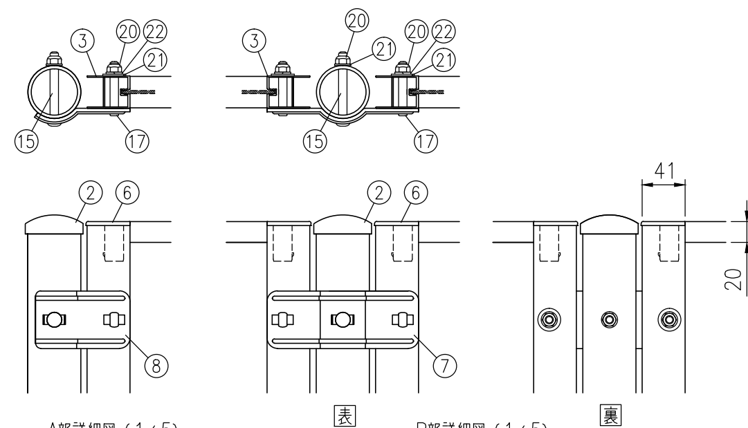
A部詳細図 (1/5)
