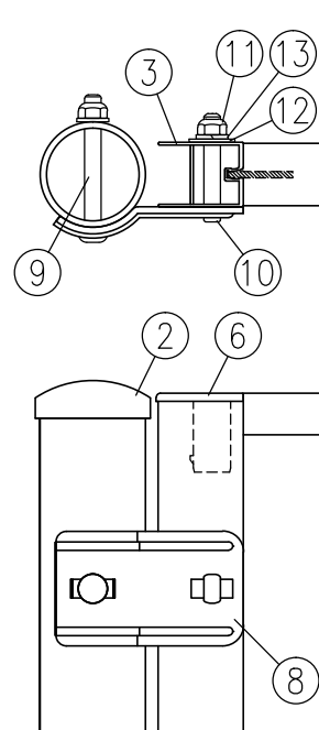
A部詳細図 (1/4)
