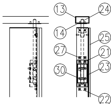
I部分詳細図 (1/10)
