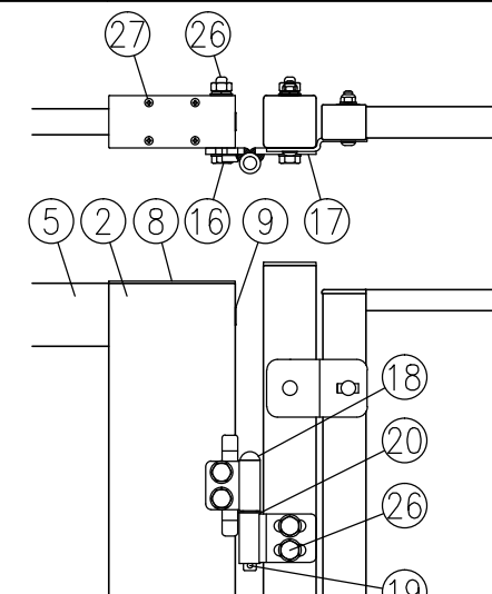
ロ部分詳細図 (1/8)
