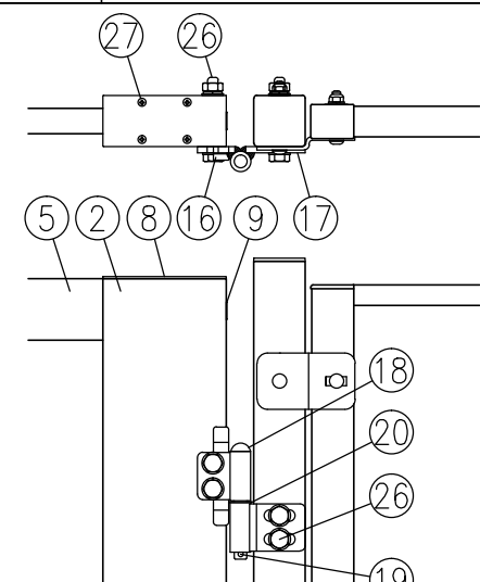
ロ部詳細図 (1/8)
