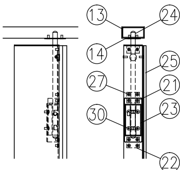
ニ部詳細図 (1/10)
