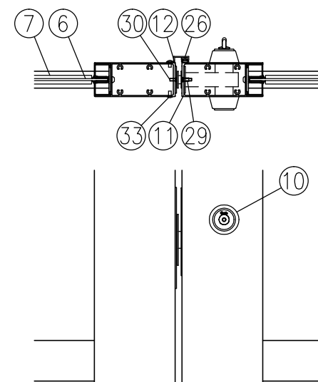
一部詳細図 (1/8)
