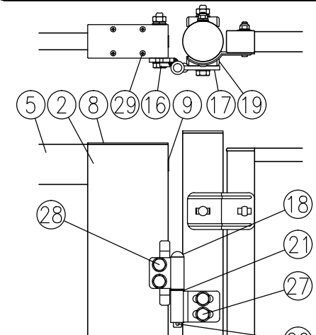
二部詳細図 (1/8)
