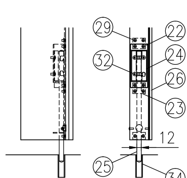
ハ部詳細図 (1/10)
