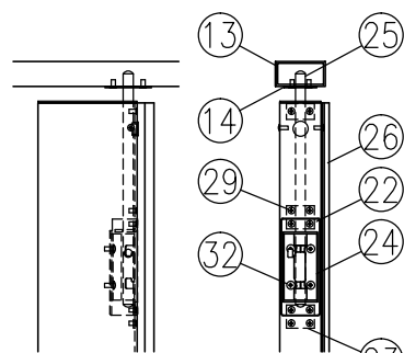
二部詳細図 (1/10)
