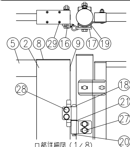
ロ部詳細図 (1/8)
