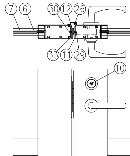
イ部詳細図 (1/8)
