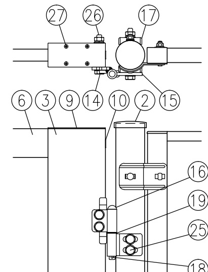
□部詳細図 (1/8)
