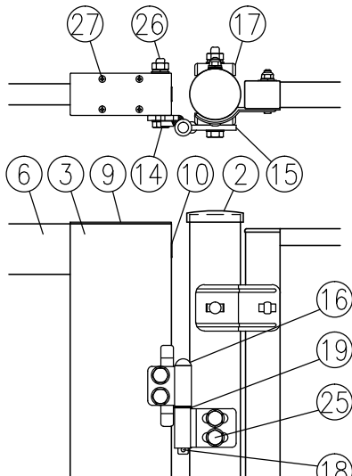
ロ部詳細図 (1/8)
