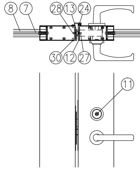
イ部詳細図 (1/8)
