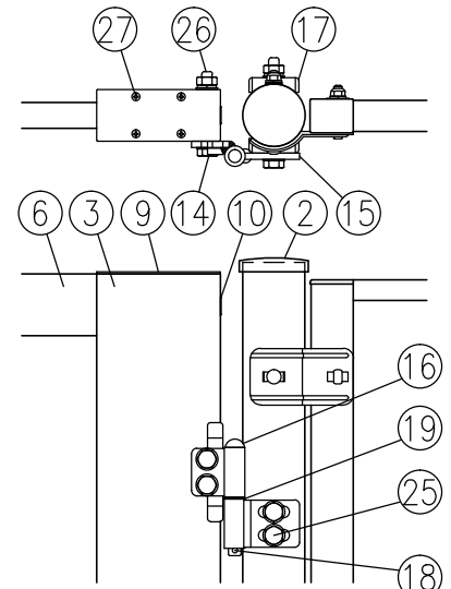
ロ部詳細図 (1/8)
