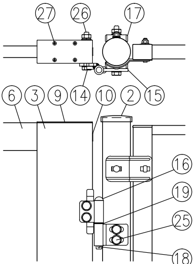
□部詳細図 (1/8)
