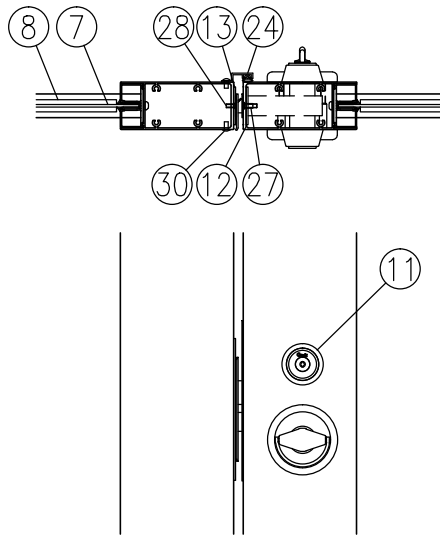
イ部詳細図 (1/8)
