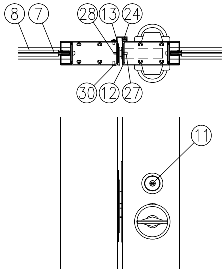
イ部詳細図 (1/8)
