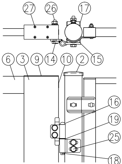
□部詳細図 (1/8)
