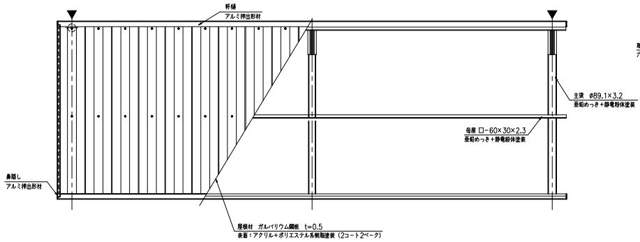
正面図 (S=1:20)
