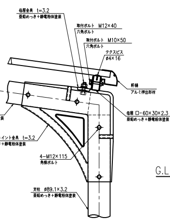
B部詳細図 (S=1:5)
