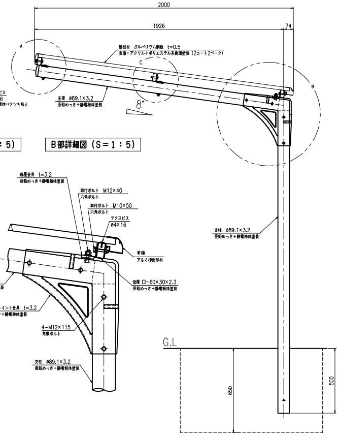
断面図 (S=1:10)
