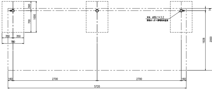
平面図 (S=1:20)
