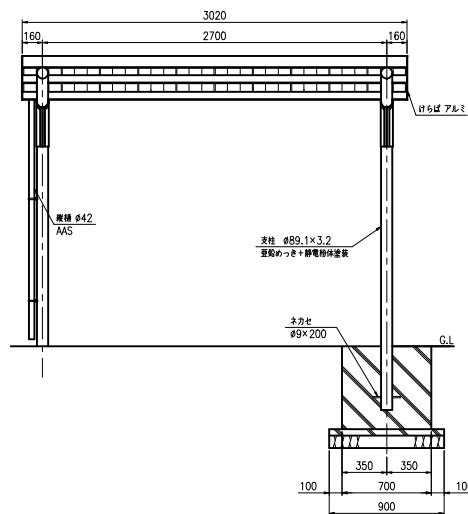
正面図 (S=1:20)
