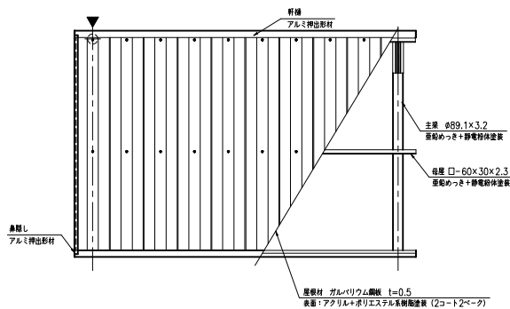
正面図 (S=1:20)
