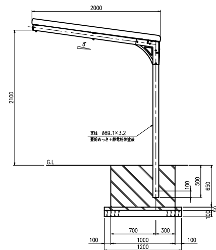
側面図 (S=1:20)
