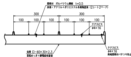
屋根材取付詳細図 (S=1:5)
