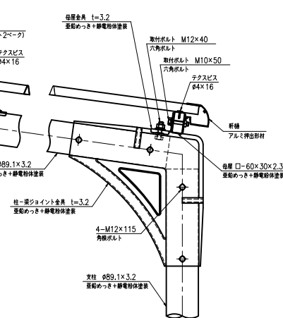
C部詳細図 (S=1:5)
