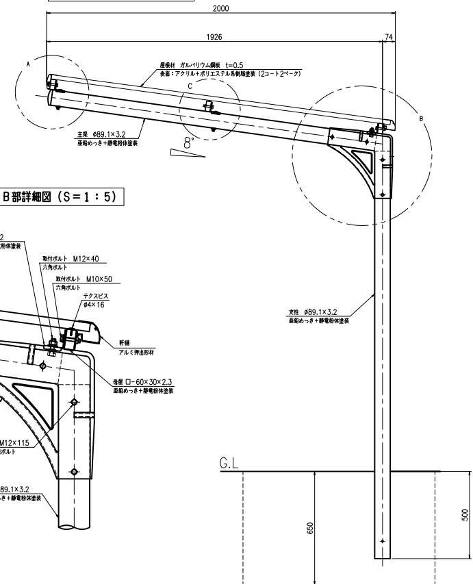
断面図 (S=1:10)
