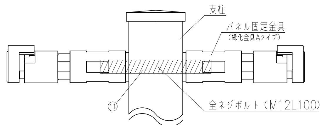
A部詳細図
