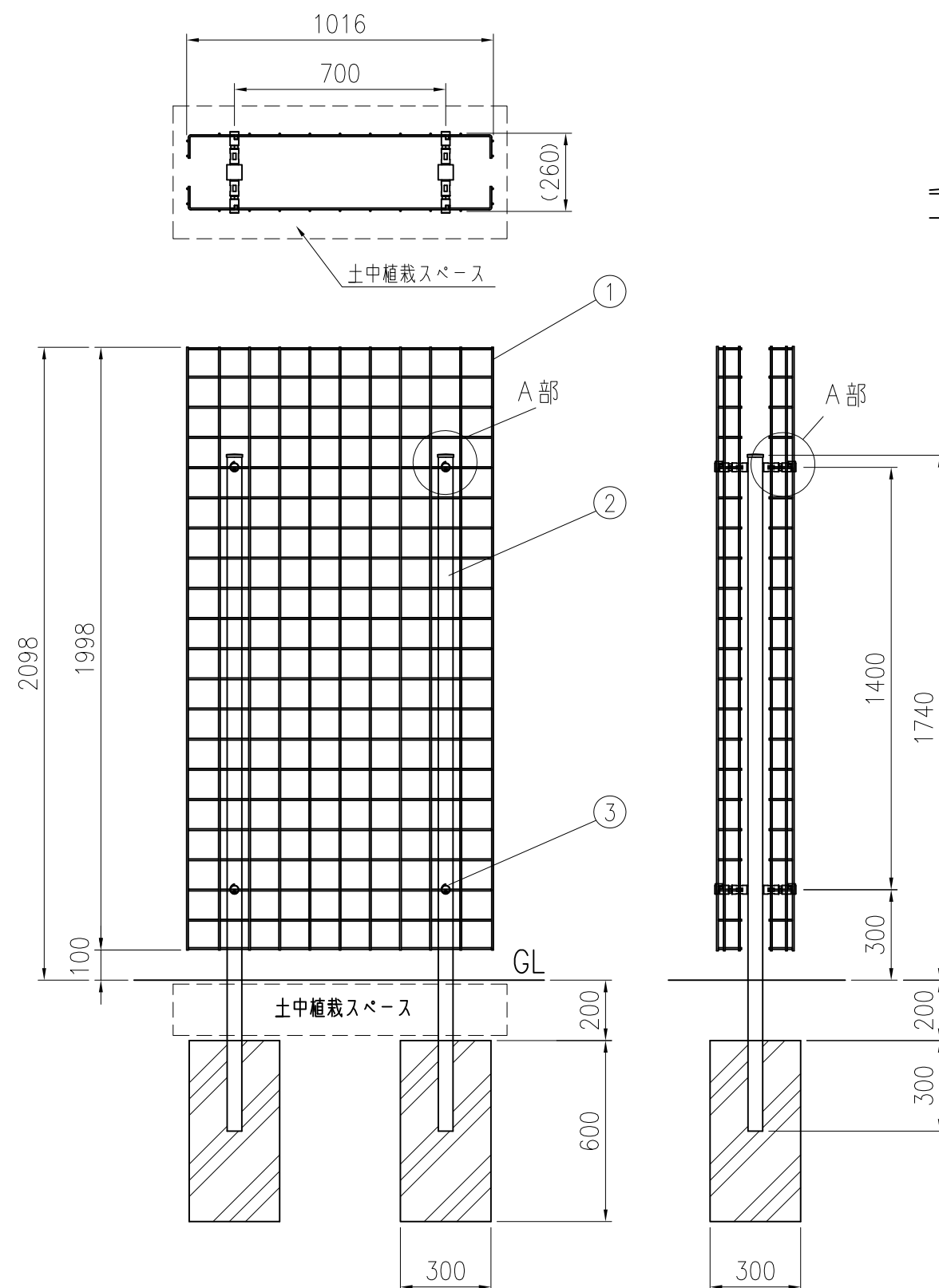
組立図
