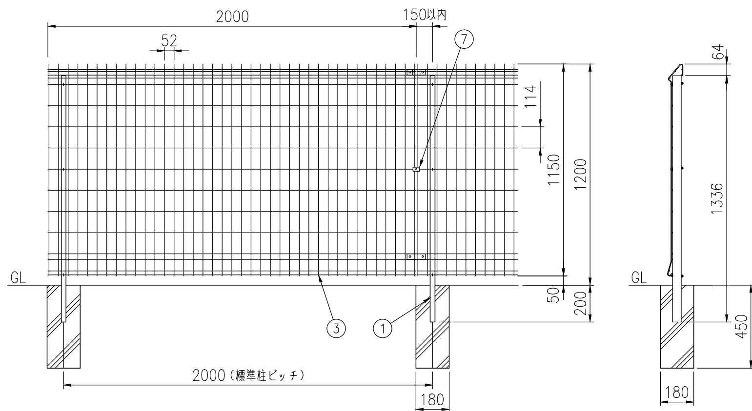
組立図 (1/20) 注) 基礎の大きさは参考寸法です。
