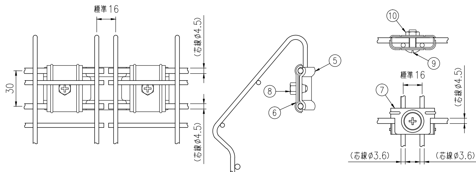
パネル止金具詳細図 (1/2) 注) パネル止金具の取付けは、逆方向(内側)からでもできます。
