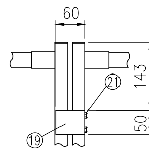
ヘ部詳細図 (1/8)
