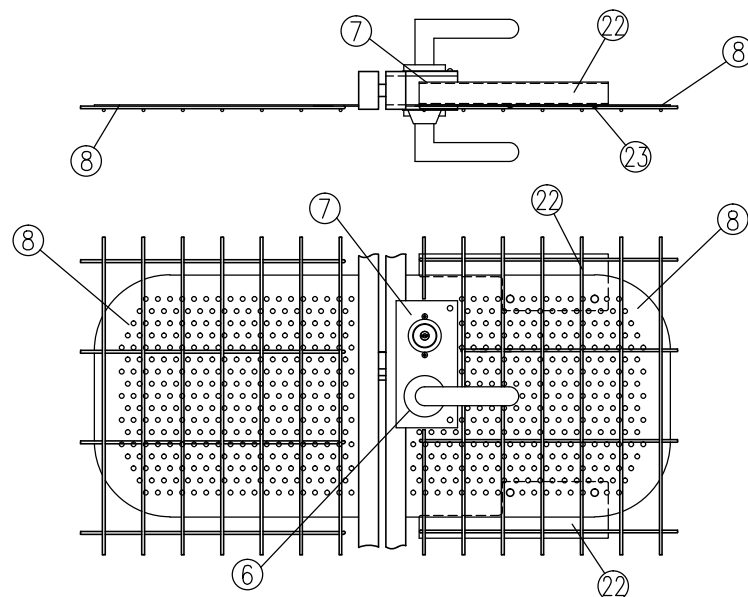
イ部詳細図 (1/10)
