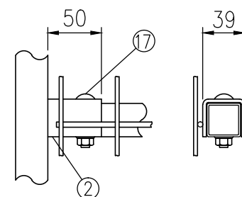
ホ部詳細図 (1/5)
