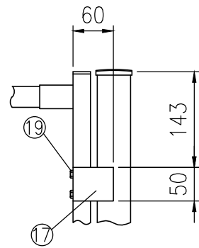
ホ部詳細図 (1/8)
