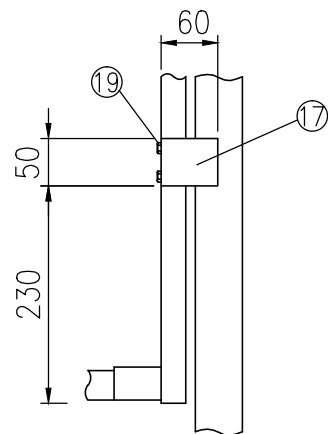
へ部詳細図 (1/8)
