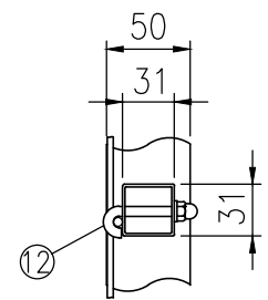
ハ部詳細図 (1/5)
