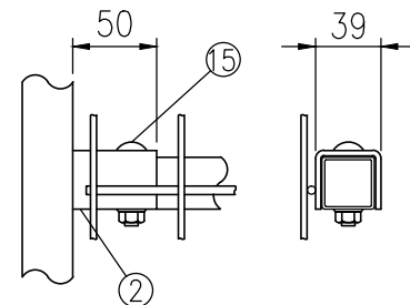
ニ部詳細図 (1/5)
