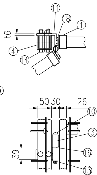
ロ部詳細図 (1/8)
