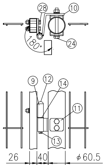
イ部詳細図 (1/8)
