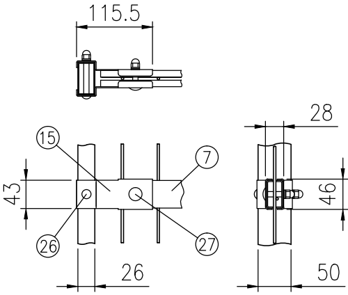
ロ部詳細図 (1/8)
