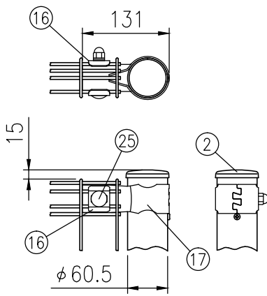
ハ部詳細図 (1/8)
