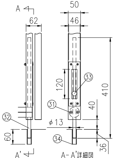
ヘ部詳細図 (1/8)
