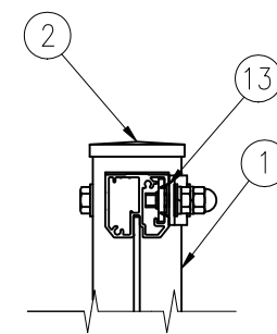
D部 詳細図 (1/5)
