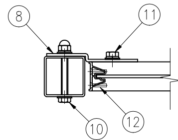
A-A 断面図 (1/5)
