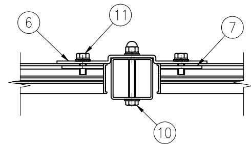
B-B 断面図 (1/5)
