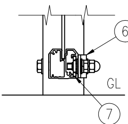
E部 詳細図 (1/5)
