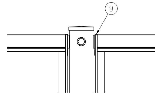
C部 詳細図 (1/5)
