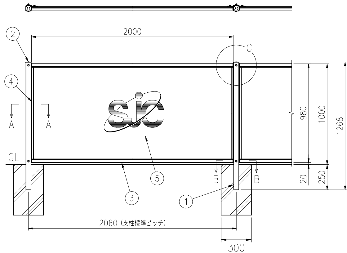
組立図 (1/25)
