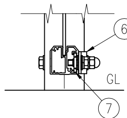
E部 詳細図 (1/5)
