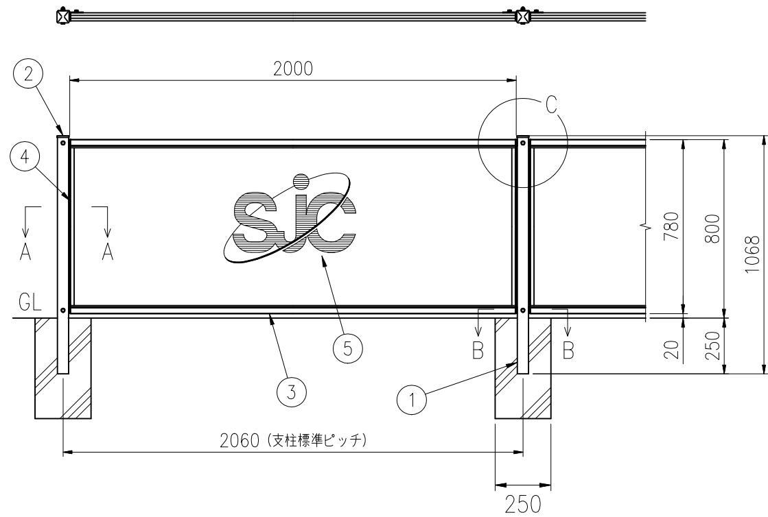
組立図 (1/25)
