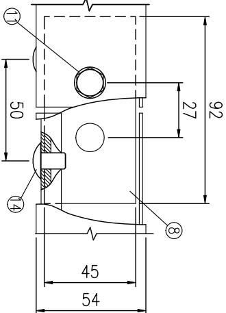
接統部詳細図 (1/2)
