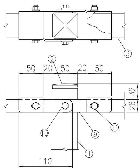
取付部詳細図 (1/4)
