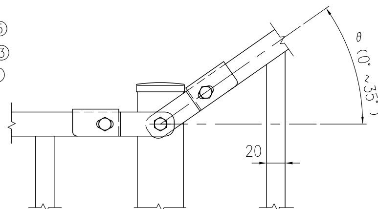
取付部詳細図 (1/4)
