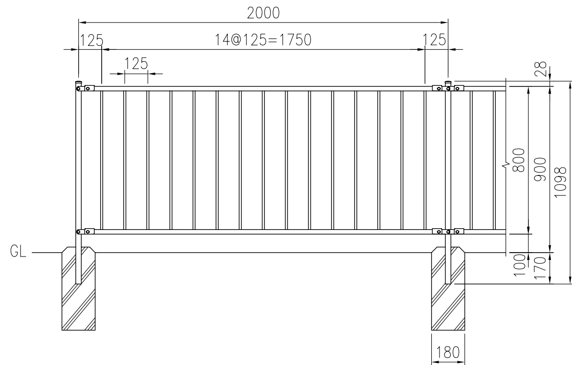
組立図 (1/20)
