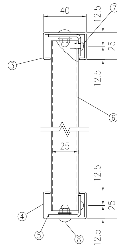
注) 下横棧には水抜穴(4カ所)があいてあります。 フェンス組立詳細図 (1/2)
