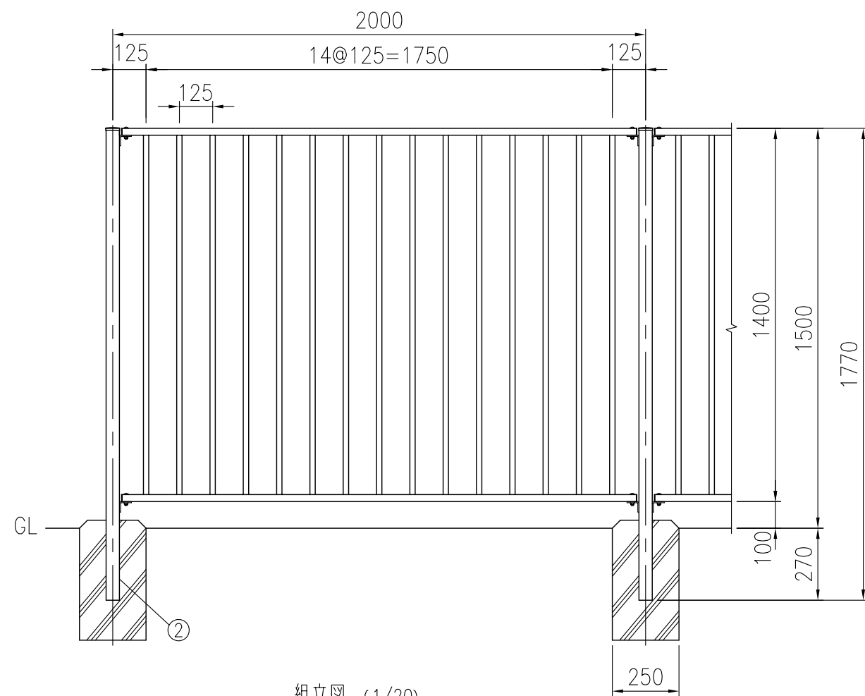
組立図 (1/20)
