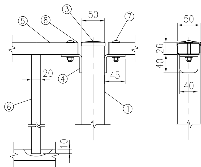
取付部詳細図 (1/5)
