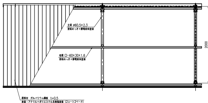
正面図 (S=1:20)
