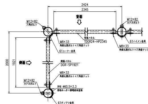
パネル取付詳細図 (S=1:5)
