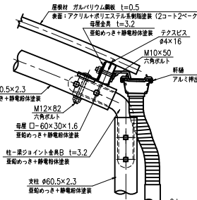
D部詳細図 (S=1:5)
