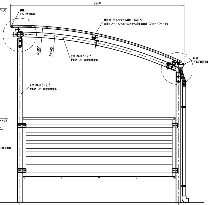
A-A断面図 (S=1:10)
