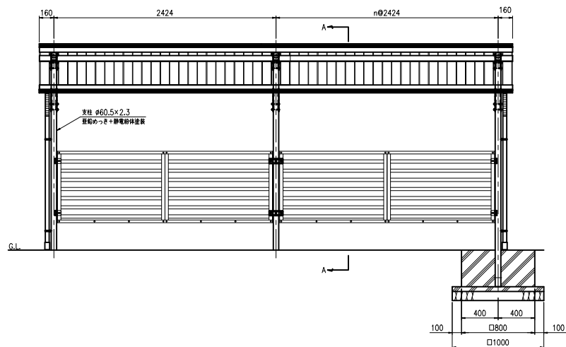
正面図 (S=1:20)
