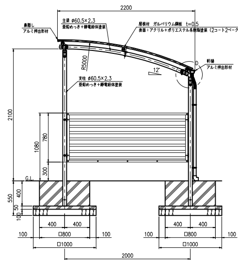
側面図 (S=1:20)
