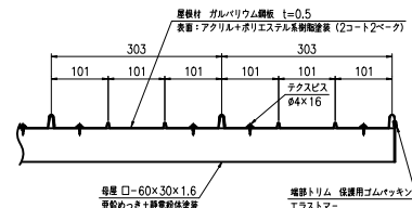
屋根材取付詳細図 (S=1:5)
