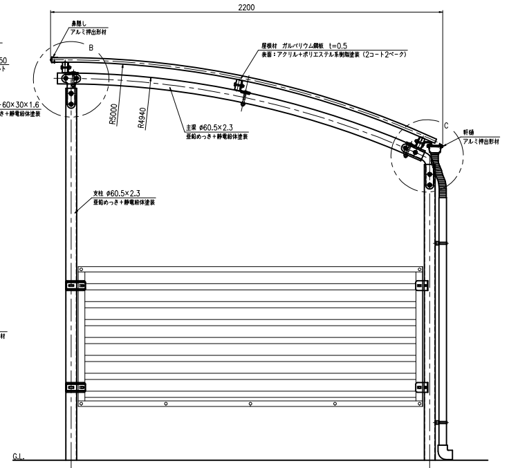
A-A断面図 (S=1:10)
