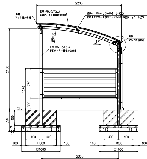
側面図 (S=1:20)
