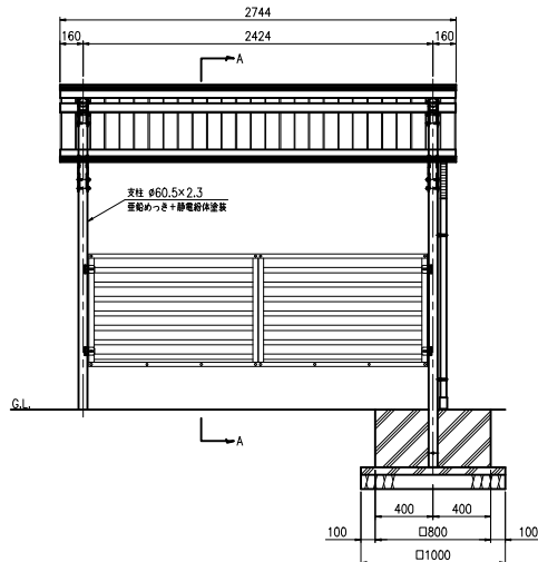
正面図 (S=1:20)
