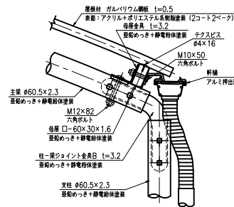
D部詳細図 (S=1:5)
