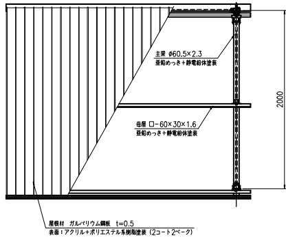
平面図 (S=1:20)
