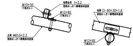
母屋取付詳細図 (S=1:5)
