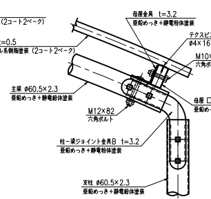
D部詳細図 (S=1:5)
