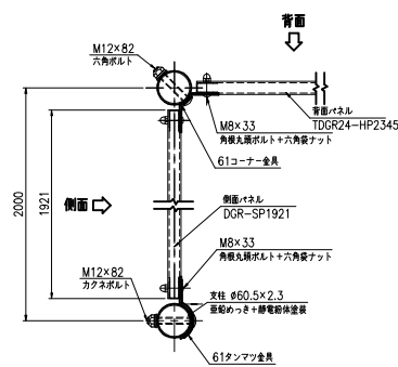
パネル取付詳細図 (S=1:5)
