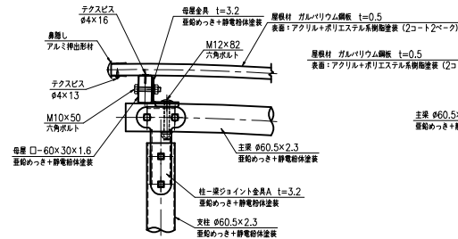
B部詳細図 (S=1:5)
